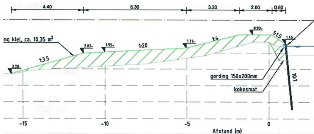
Figuur 2 Dwarsprofiel van dijkversterking (concept)
